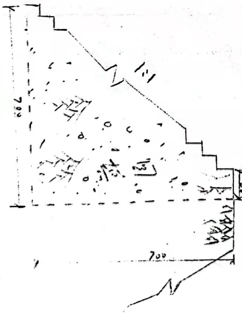
四 边坡支护图
